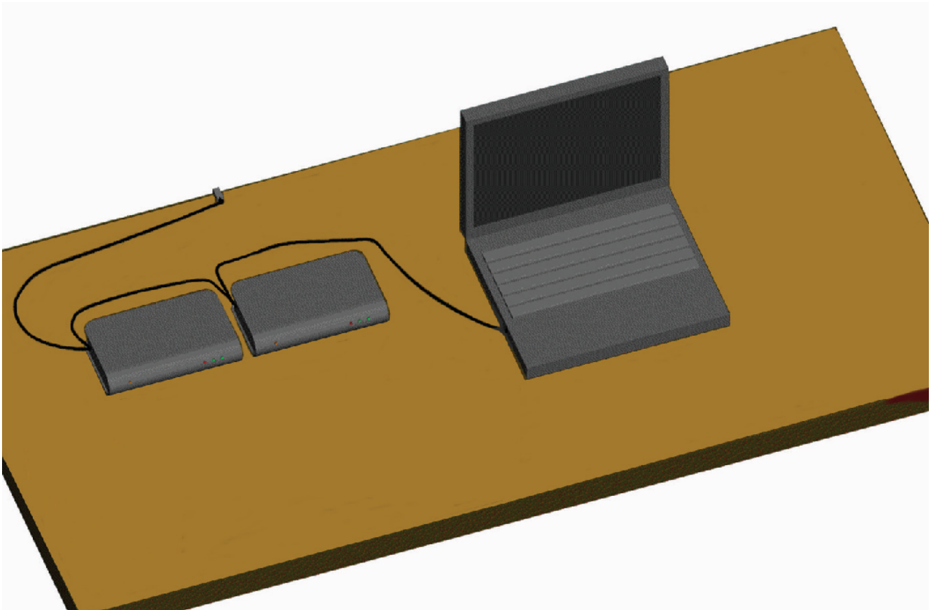
WYG-it Watcher
