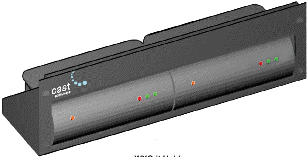
WYG-it Holder
