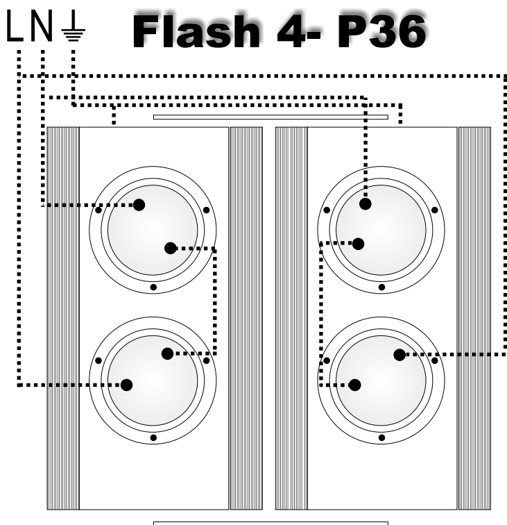
LAMP P36 120V 650 W
